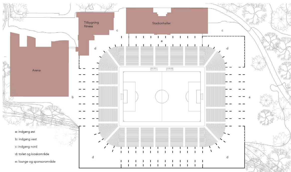
Illustrationer: Johan Thomas Buus Snit og plan for forslag til nyt stadion
