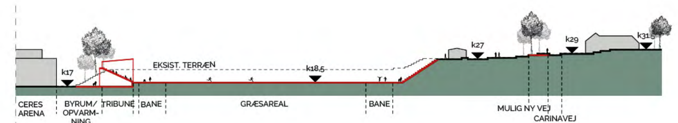
Principsnit BB - Tværsnit af atletikstadion
