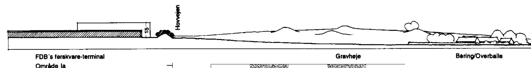
Snit B-B
